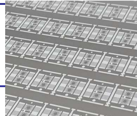
ドライフィルムレジスト による加工例
